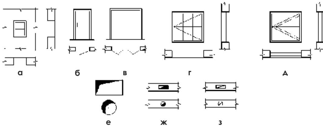
Рис. 100 - Умовні позначення елементів будинків:
