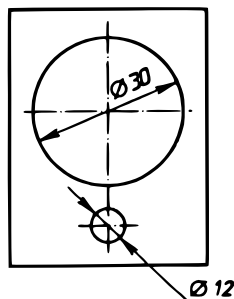
Рис. 36 - Позначення розміру діаметра
