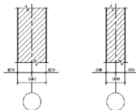
Рис. 106 - Прив'язка до координатних осей: а - зовнішніх несучих стін; б - внутрішніх несучих стін
