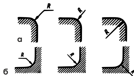
Рис. 42 - Нанесення розмірів радіусів заокруглень: а – зовнішніх; б – внутрішніх
