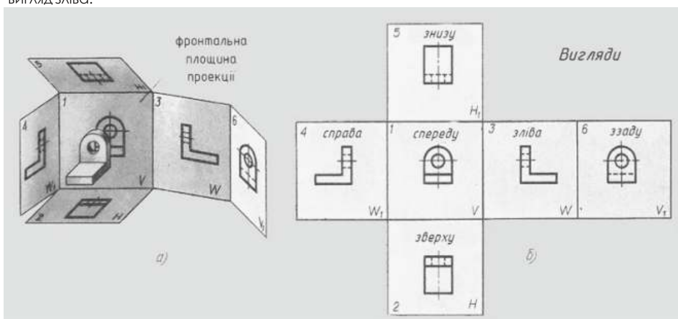
Рис. 57 - Вигляди
