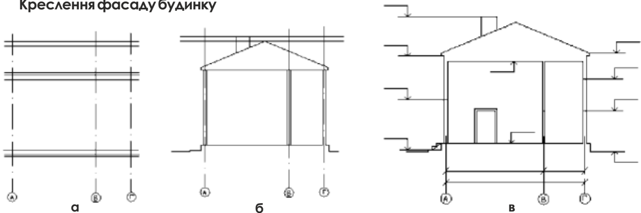
Рис. 107 - Послідовність виконання креслення розрізу будинку (а, б, в)
