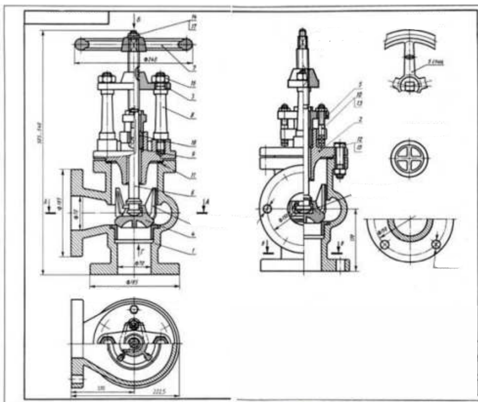
Рис. 123 - Складальне креслення виробу
