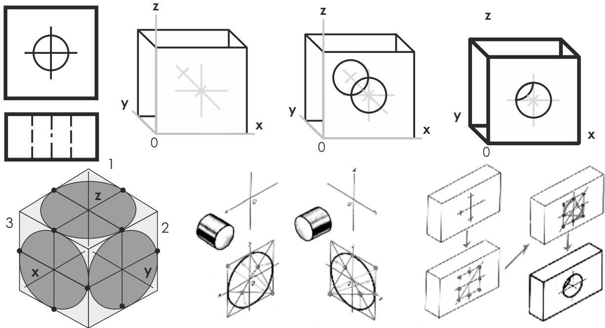
Побудова диметричної аксонометрії деталі з круглим наскрізним отвором.
