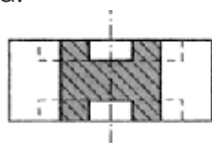
Рис. 71 - Накладений переріз
