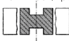
Рис. 72 - Винесений переріз в розриві
