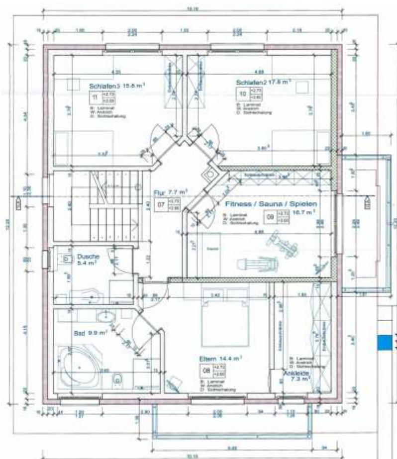
Рис. 119 - План III поверху, масштаб 1:50
