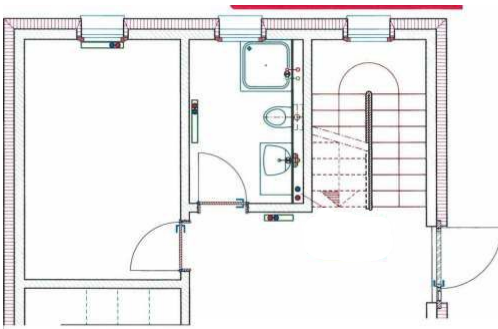
Рис. 111 - Схема розташування труб гарячої та холодної води на плані поверху
