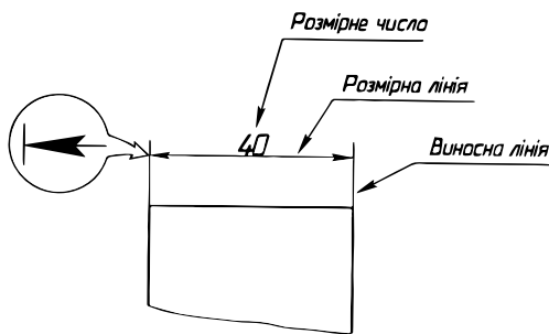
Рис. 21 - Елементи лінійного розміру креслення
