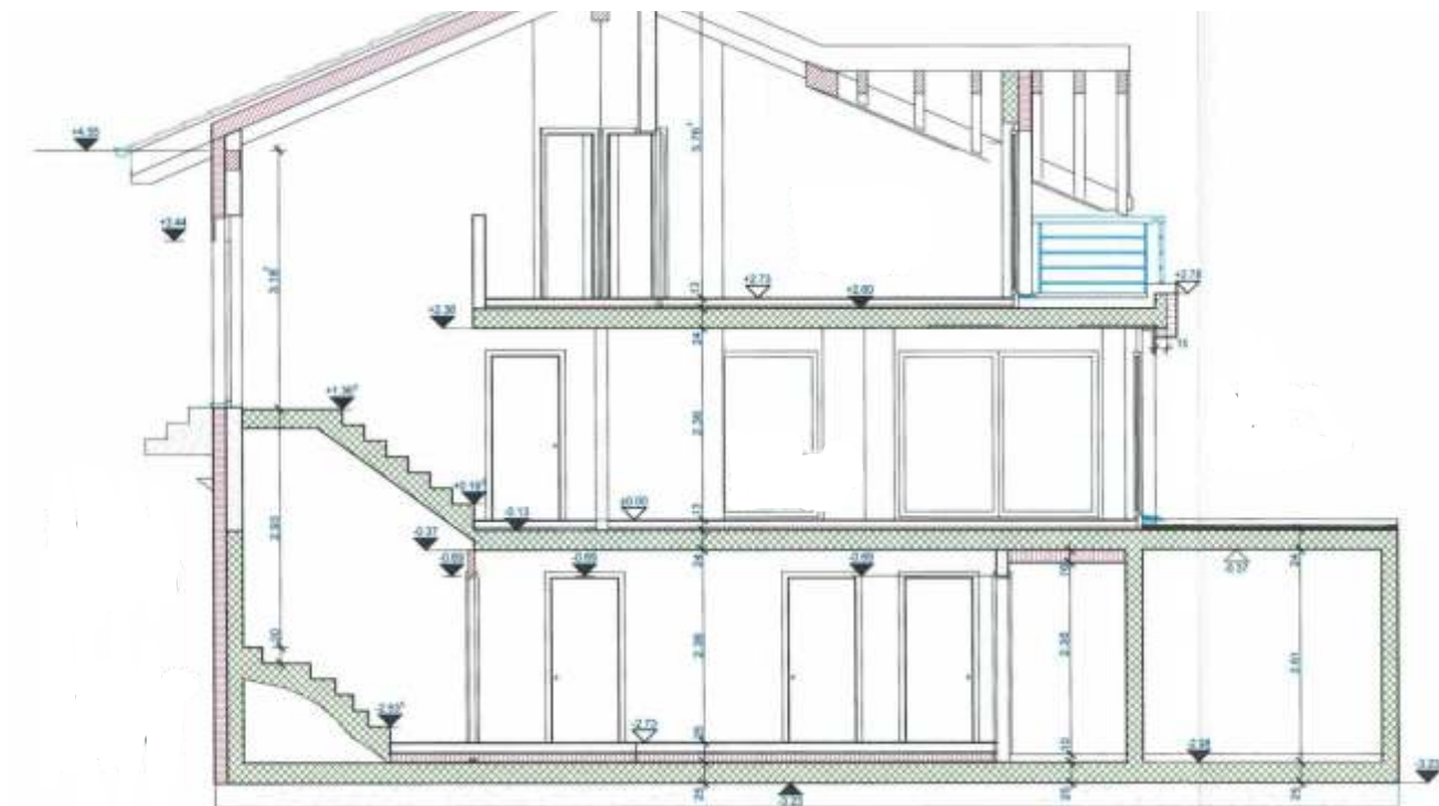
Рис. 120 - Розріз будівлі
