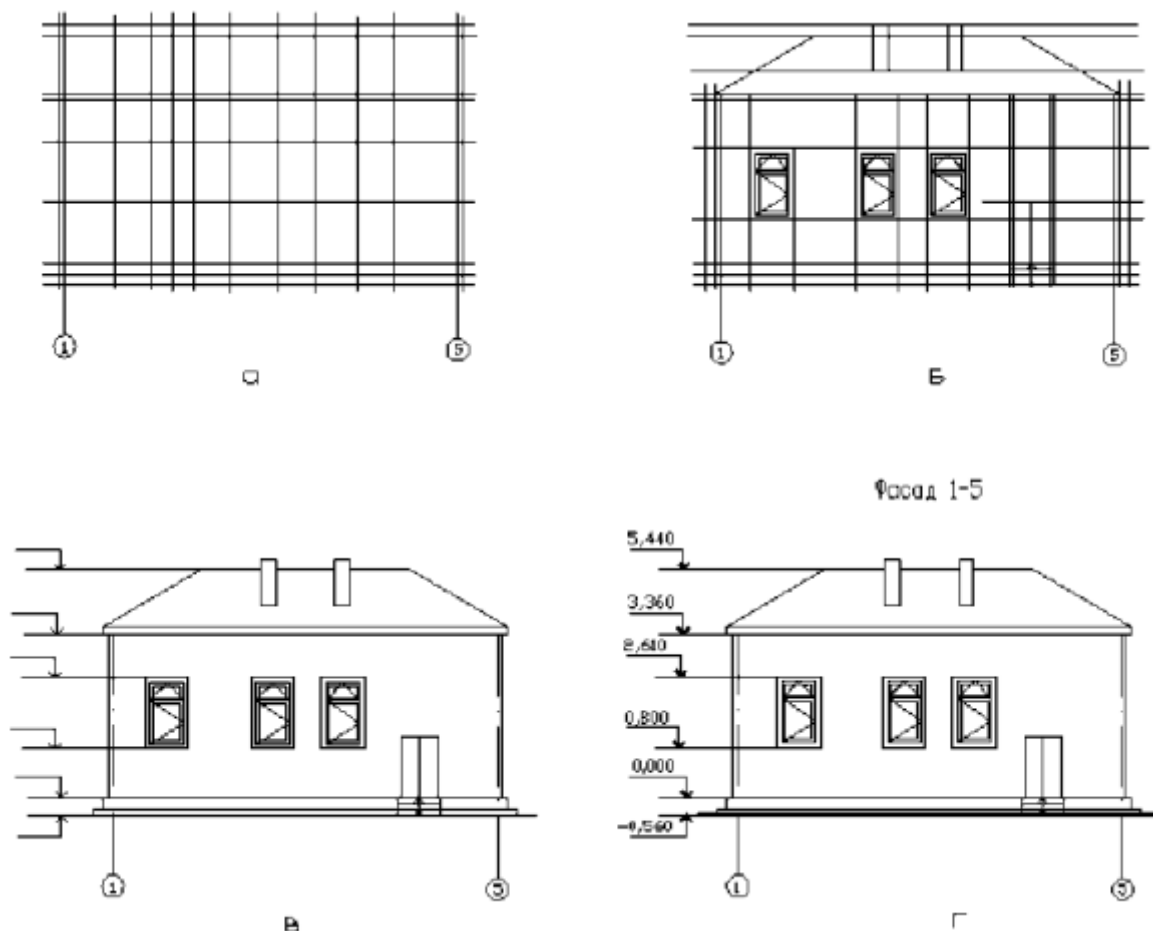
Рис. 108 - Послідовність виконання креслення фасаду будинку
