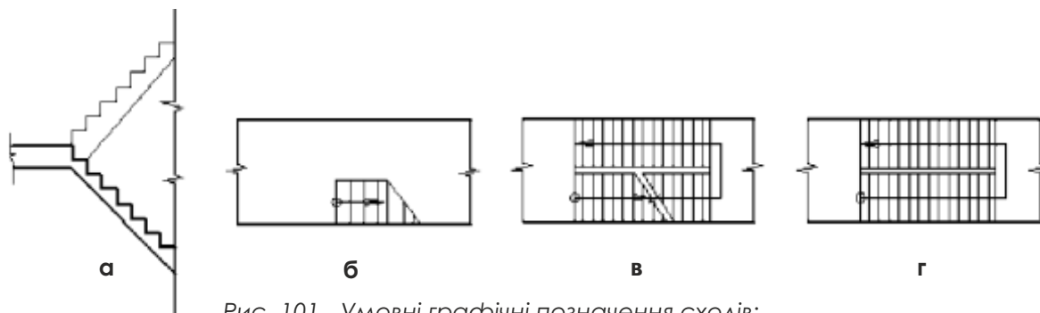
Рис. 101 - Умовні графічні позначення сходів:
