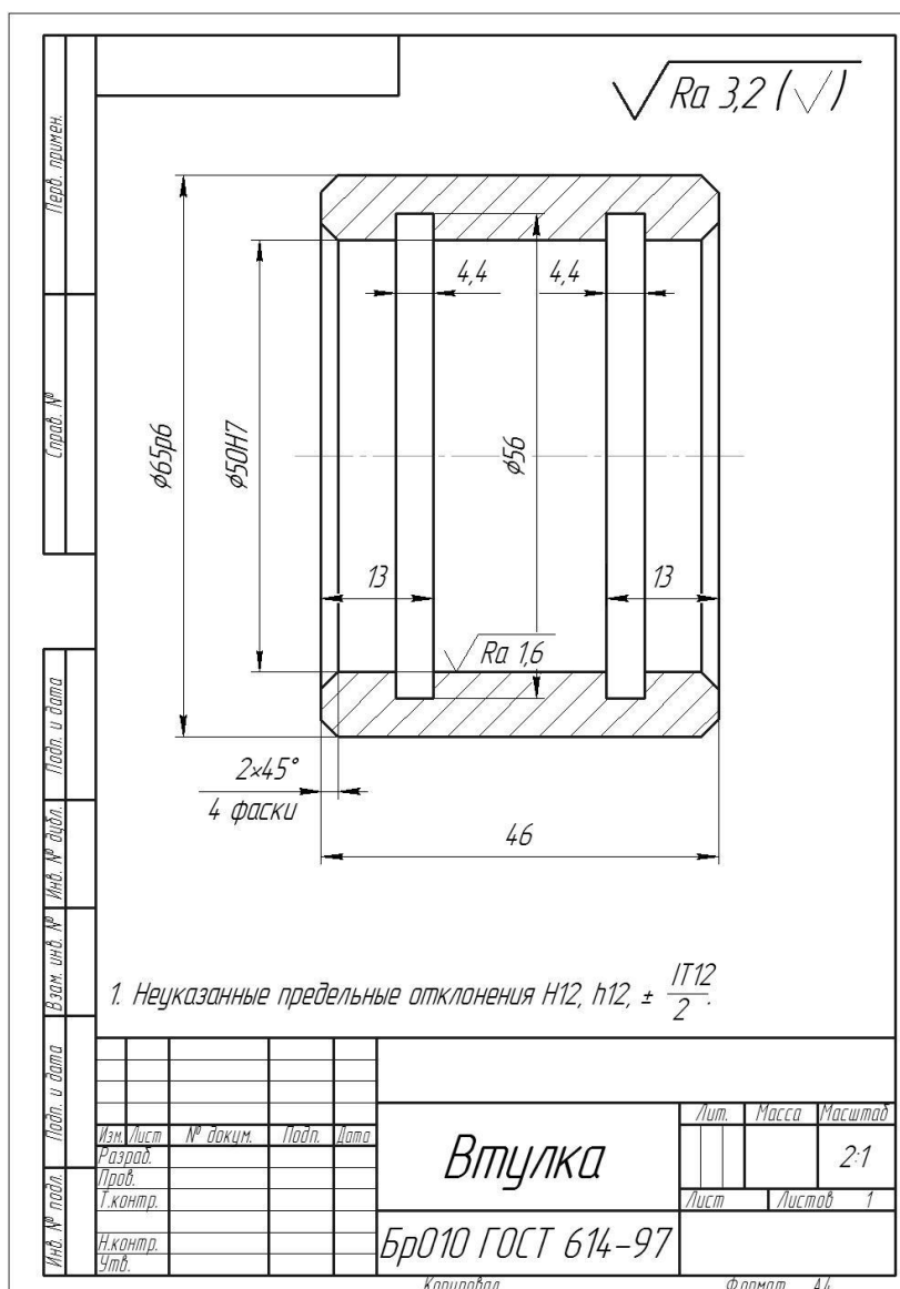
Рисунок 1– Креслення деталі
