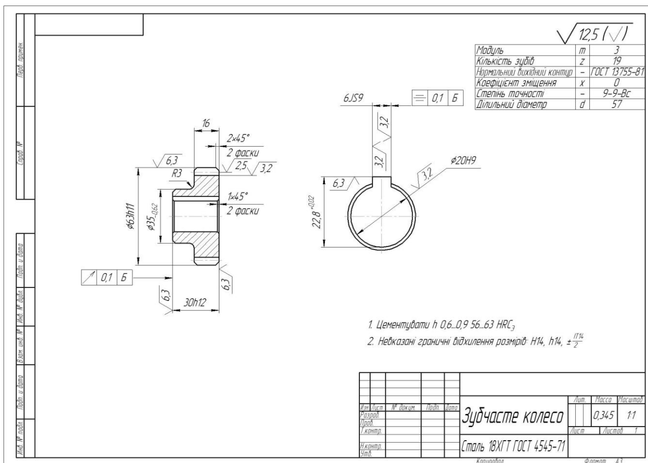
Рисунок 1— Креслення деталі
