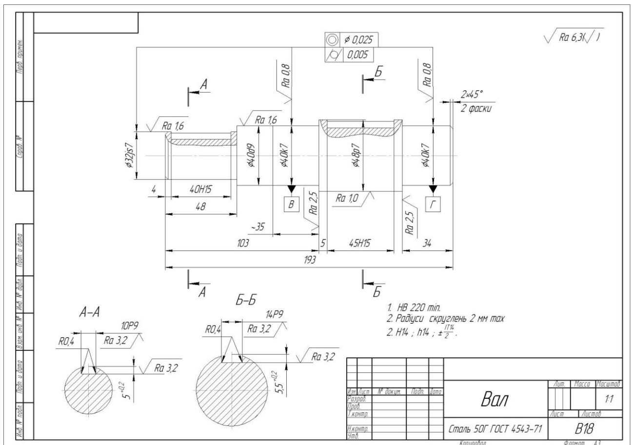
Рисунок 1– Креслення деталі
